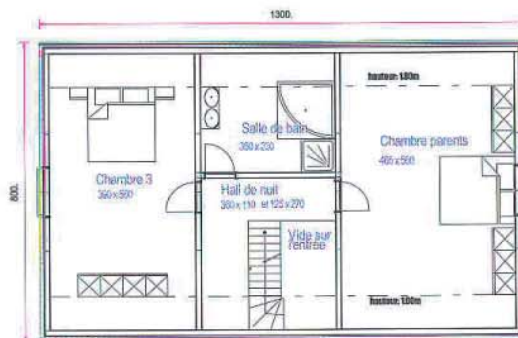
Plan Etage
