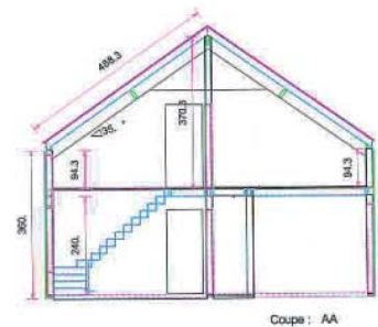
Coupe : AA
