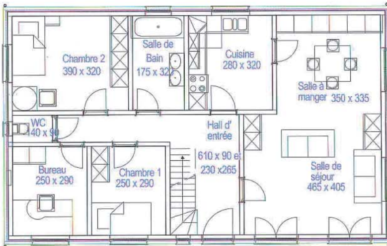
Plan Rez de Chaussée
