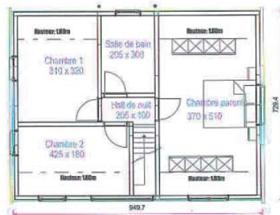
Plan Etage
