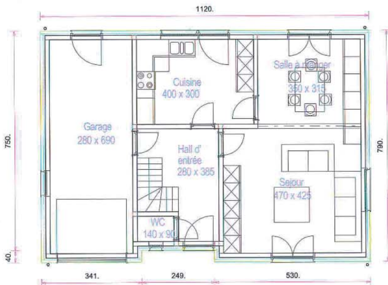
Plan Rez de Chaussée
