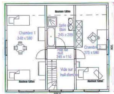
Plan Etage
