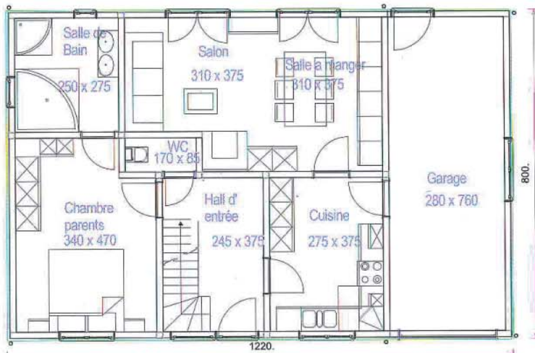
Plan Rez de Chaussée
